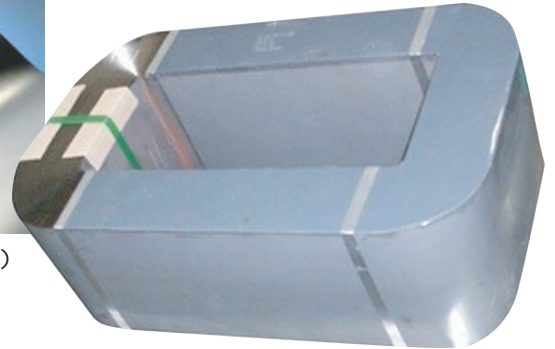
Lõi vô định hình (Lõi Amorphous)
